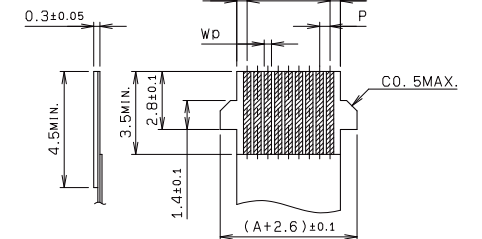
適用 Au FFC 寸法 APPLICABLE Au FFC
