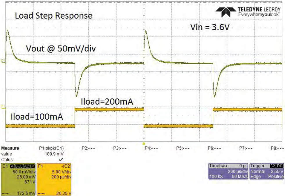
Fig 14. Load step
