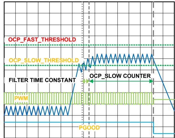
FIGURE 20. OCP_Slow
