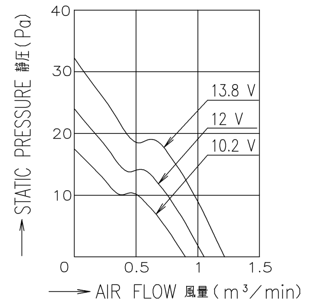
風量-静圧特性例
