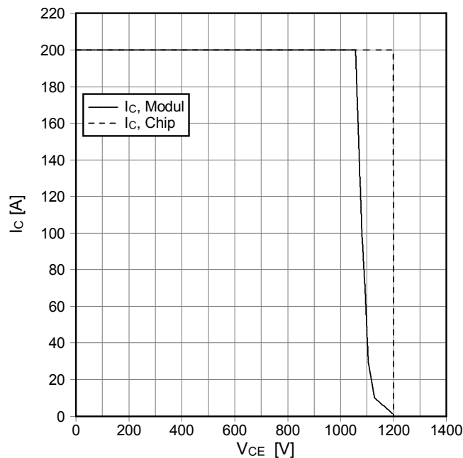
Sicherer Rückwärts-Arbeitsbereich IGBT-Wr. (RBSOA) reverse bias safe operating area IGBT-inv. (RBSOA) I_C = f(V_{CE}) V_{GE} = \pm 15\text{ V} , R_{Goff} = 1.6\ \Omega , T_{vj} = 150^\circ\text{C}
