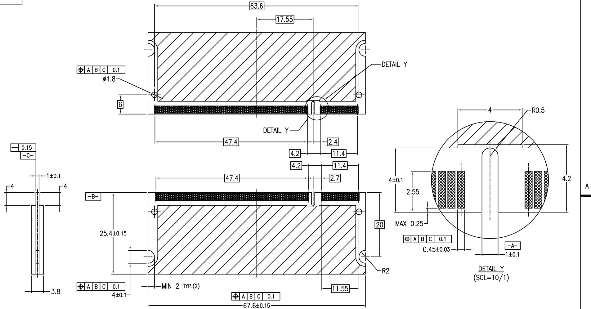
RECOMMENDED MODULE P.C.B. LAYOUT
