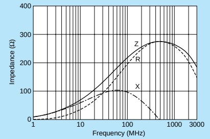
BLM18EG221SN1
