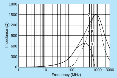
BLM18HB331SN1
