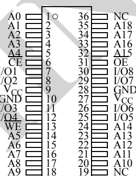
36-pin SOJ (400 mil)
