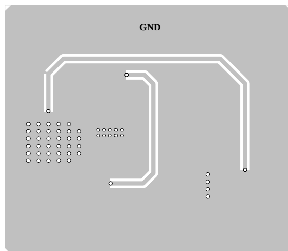
MPQ4462DQ Bottom Layer
