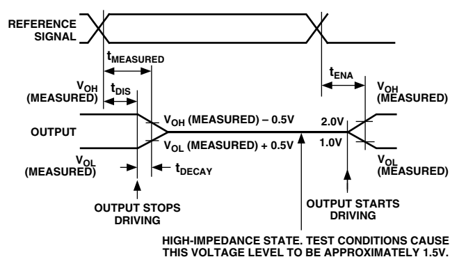
Figure 27. Output Enable/Disable
