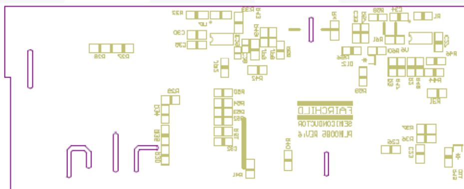
Bottom Overlay
