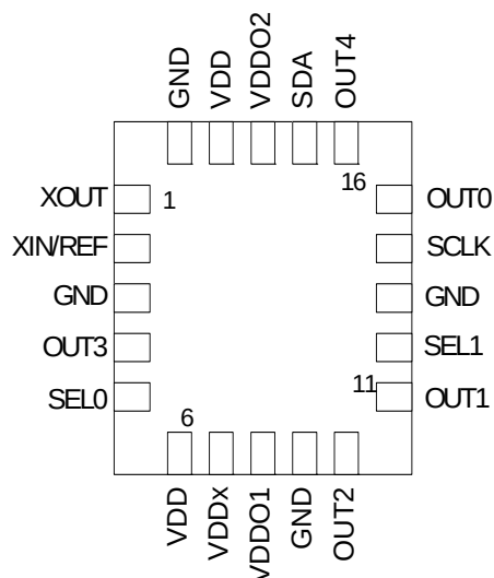
20-pin QFN
