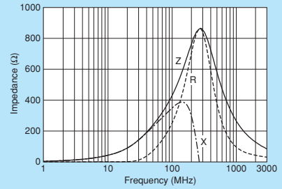
BLM18BD421SN1
