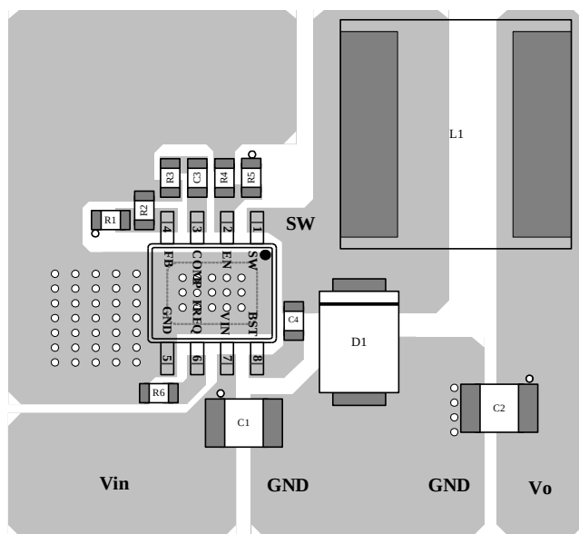
TOP Layer
