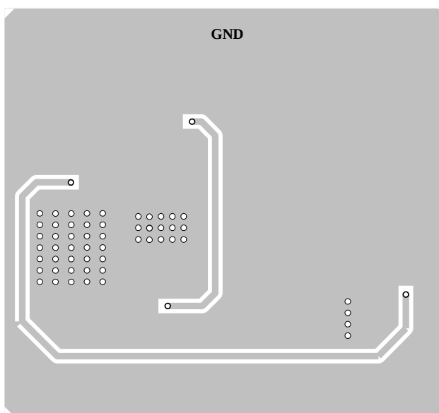
Bottom Layer
