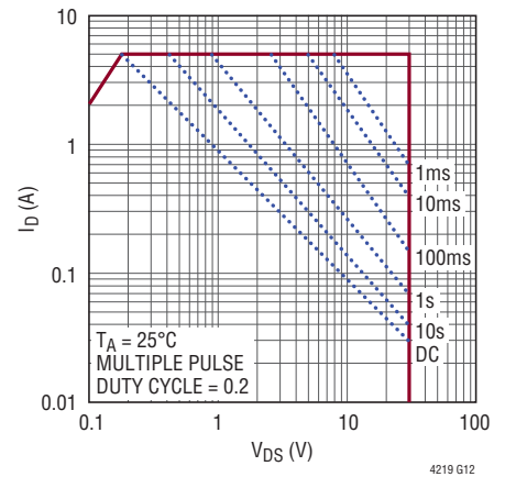
MOSFET SOA Curve
