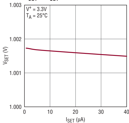
V_{SET} vs I_{SET}
