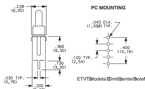
ET01MD1V3BE SPDT
