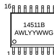
SO-16 WB
