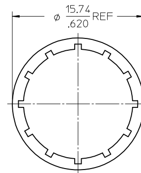
LOCKWASHER
