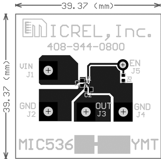
Top Layer
