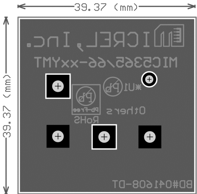
Bottom Layer
