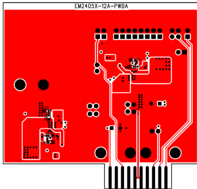
Bottom Layer
