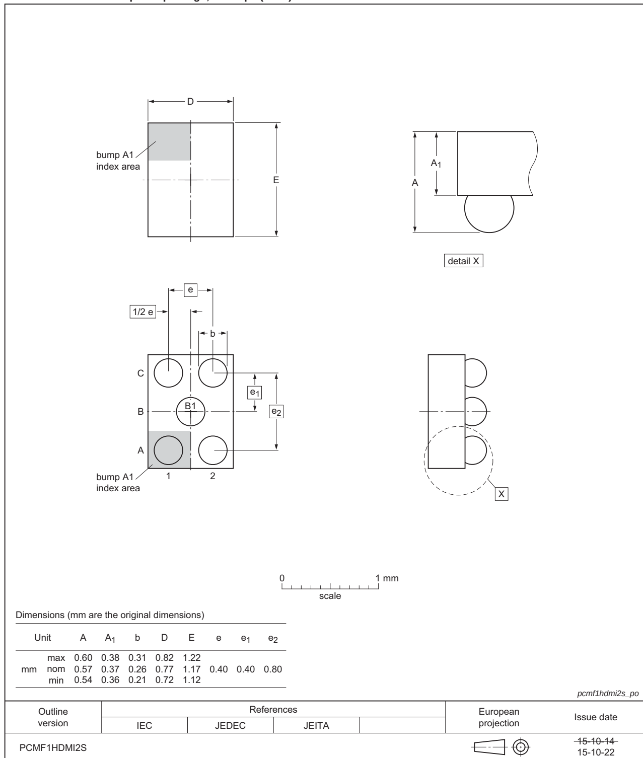
PCMF1HDMI2S
