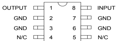
N Package (NSOIC-8)
