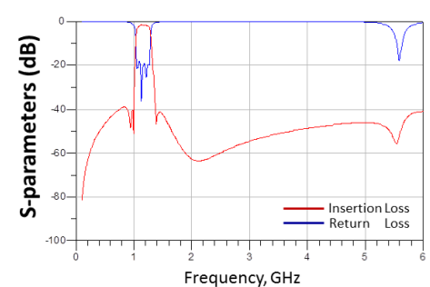
RFBPF1109B201T
