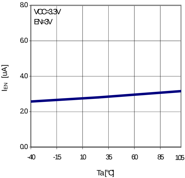
Figure 24. Ta-I EN
