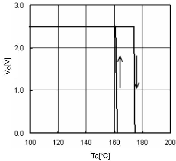
Figure 28. TSD
