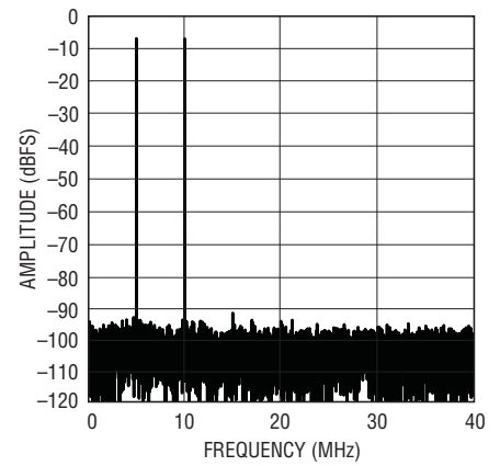
LTC2259-12: 8k Point 2-Tone FFT, f_{IN} = 70\text{MHz} , 75\text{MHz} , -1\text{dBFS} , 80\text{Mps}
