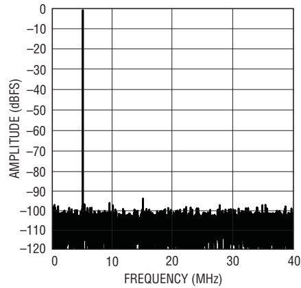
LTC2259-12: 8k Point FFT, f_{IN} = 5\text{MHz} , -1\text{dBFS} , 80\text{Mps}
