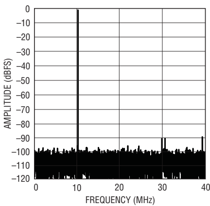
LTC2259-12: 8k Point FFT, f_{IN} = 70\text{MHz} , -1\text{dBFS} , 80\text{Mps}
