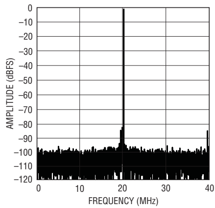
LTC2259-12: 8k Point FFT, f_{IN} = 140\text{MHz} , -1\text{dBFS} , 80\text{Mps}
