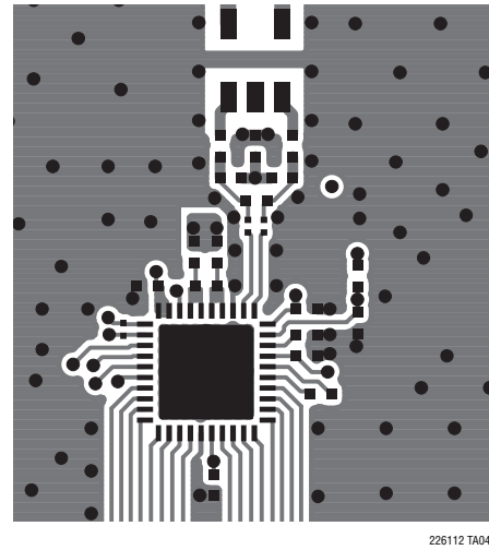
Top Side
