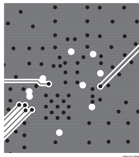
Inner Layer 3
