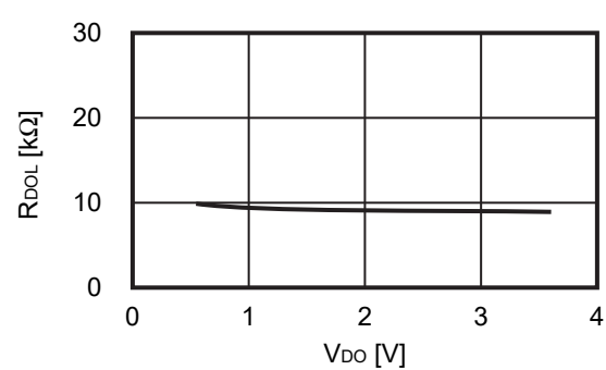
3.4 R_{DOL} vs. V_{DO}
