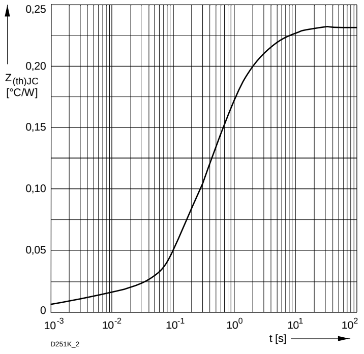
Bild / Fig. 7 Transient innerer Wärmewiderstand Transient thermal impedance Z_{thJC} = f(t) , DC 1 - Beidseitige Kühlung / Two-sided cooling 2 - Anodenseitige Kühlung / Anode-sided cooling 3 - Kathodenseitige Kühlung / Cathode-sided cooling
