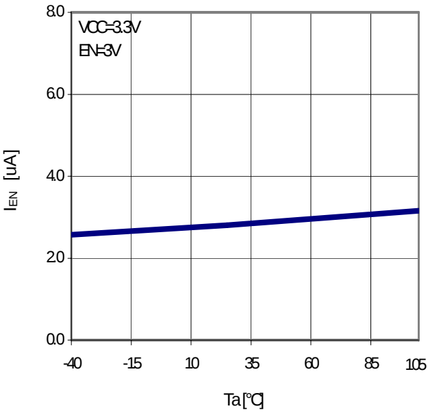
Fig.24 T_a - I_{EN}
