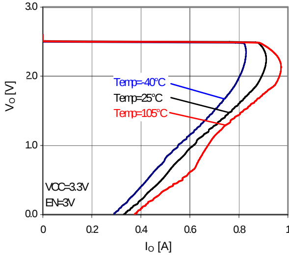
Fig.29 OCP
