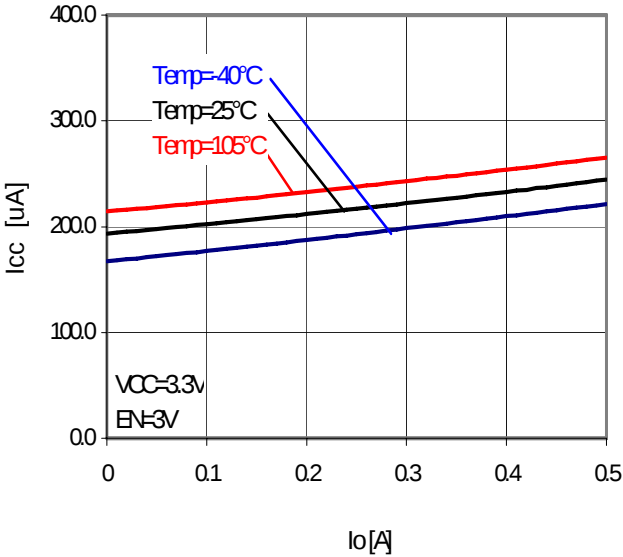
Fig.30 I_o-I_{cc}
