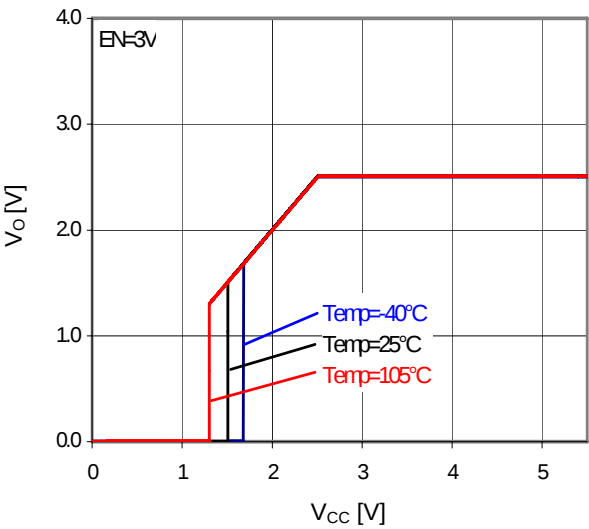
Fig.27 V_{cc}-V_o ( I_o=0mA )
