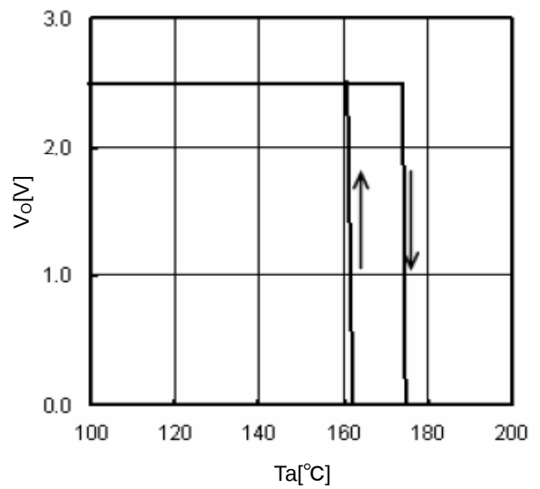
Fig.28 TSD
