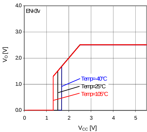
Fig.27 V_{CC}-V_O ( I_O=0mA )
