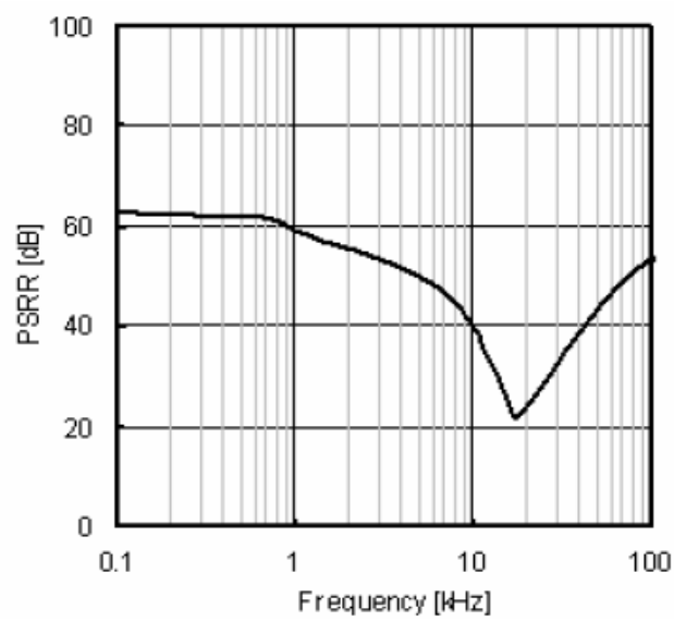
Fig.32 PSRR ( I_o=0 mA)
