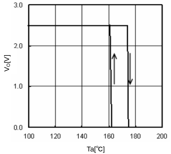
Fig.28 TSD
