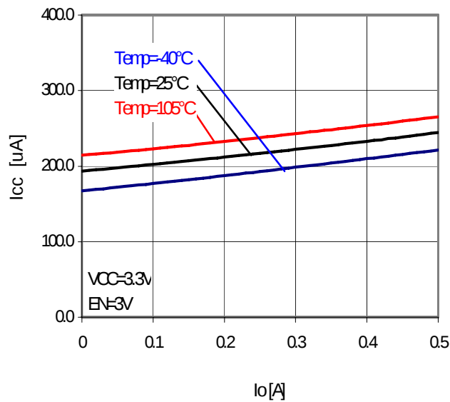
Fig.30 I_o-I_{cc}
