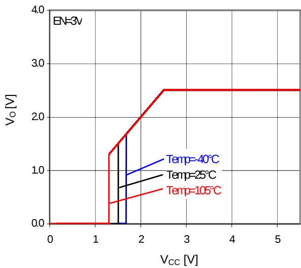
Fig.27 V_{cc}-V_o ( I_o=0mA )
