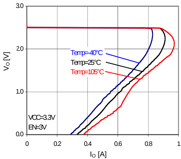
Fig.29 OCP
