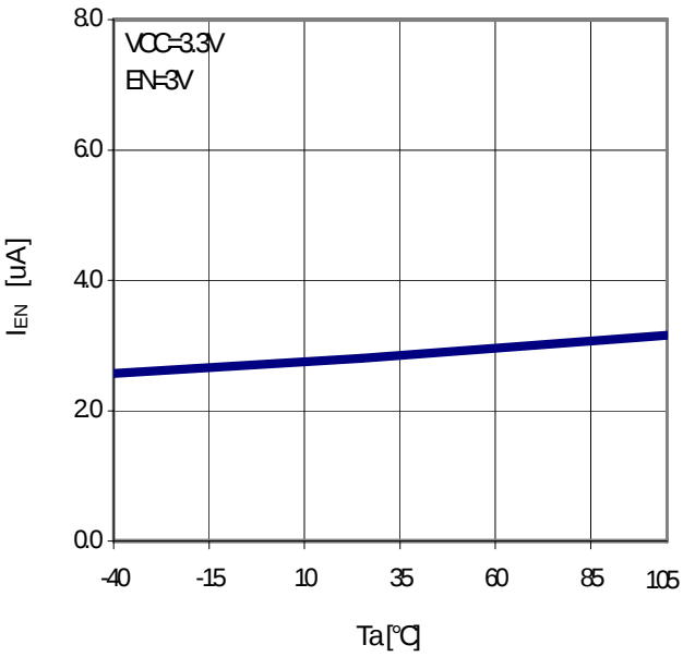
Fig.24 T_a - I_{EN}
