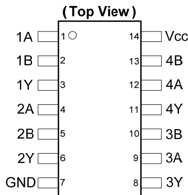
SO-14 / TSSOP-14
