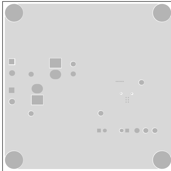
Figure 26. TPS54540-Q1EVM-593 Layer 3 Layout
