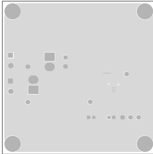
Figure 25. TPS54540-Q1EVM-593 Layer 2 Layout
