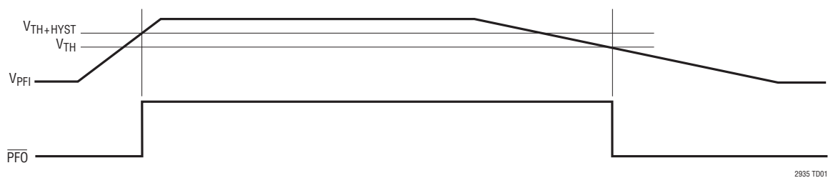
PFI/PFO Timing
