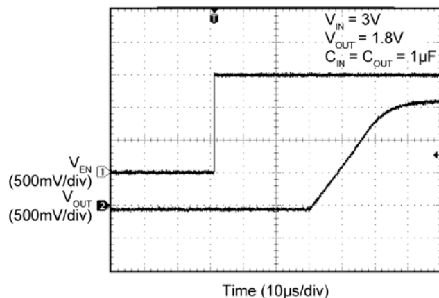
Enable Turn-On
