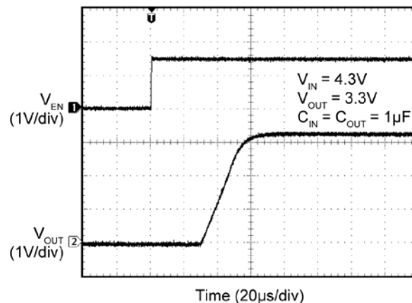
Enable Turn-On
