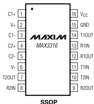
SSOP
