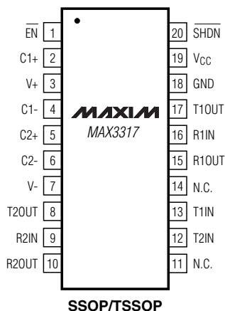
SSOP/TSSOP
