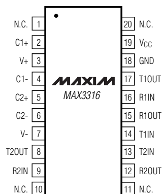
TSSOP
