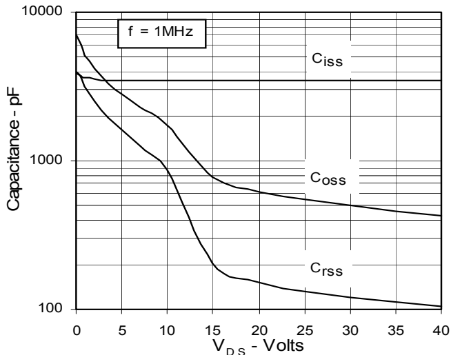
Fig. 11. Capacitance
