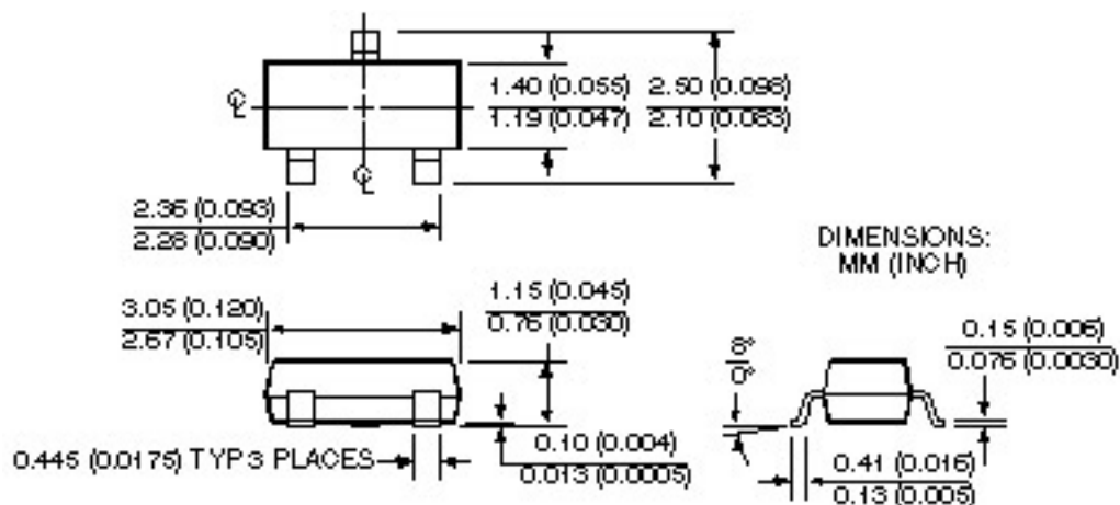
SOT-23 (M3)
