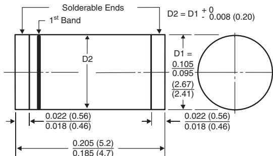
DO-213AB (GL41)
