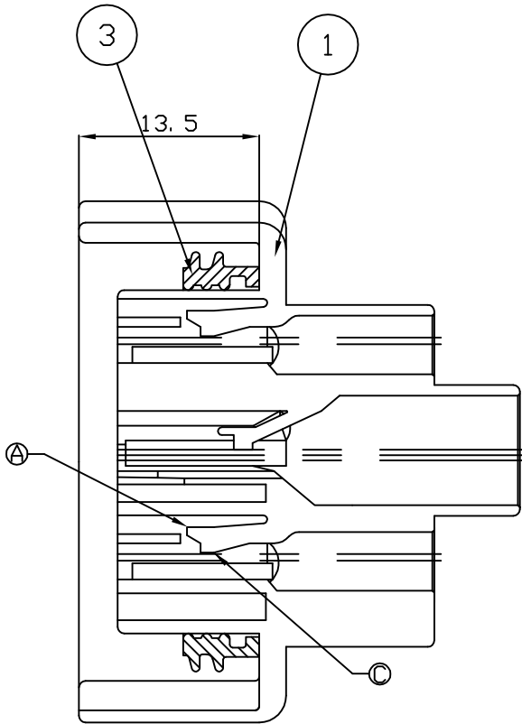
SECTION A-A
