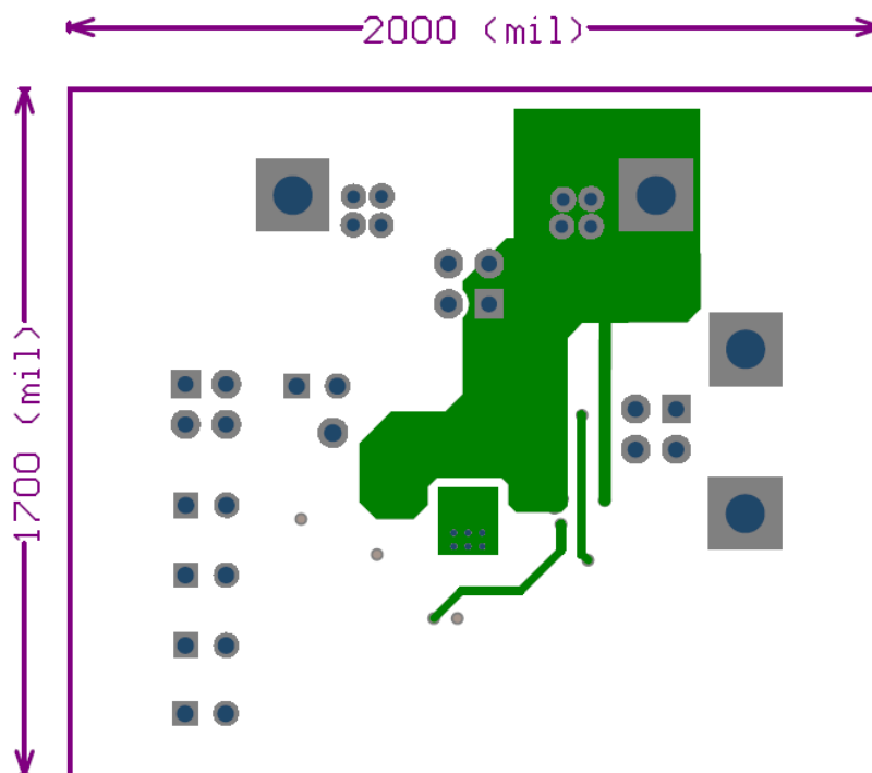
Mid Layer 2
