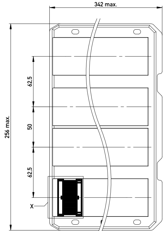
Adapterstück für board-to-board Abstand von 32mm (beidseitig verbaut mit Federleiste: 154808, Low Profile) Adapter for board-to-board height 32mm (in combination with two female connectors: 154808, low profile)
