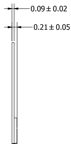
A ( 16 : 1 )
