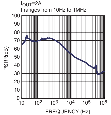
PSRR
