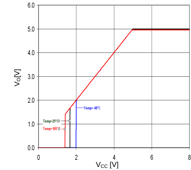
Figure 27. V_{CC} - V_O ( I_O=0\text{mA} )
