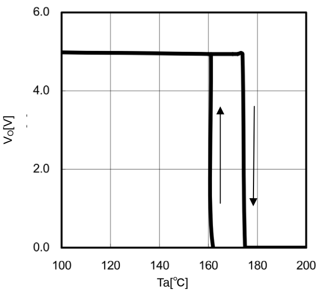
Figure 28. TSD (Io=0mA)
