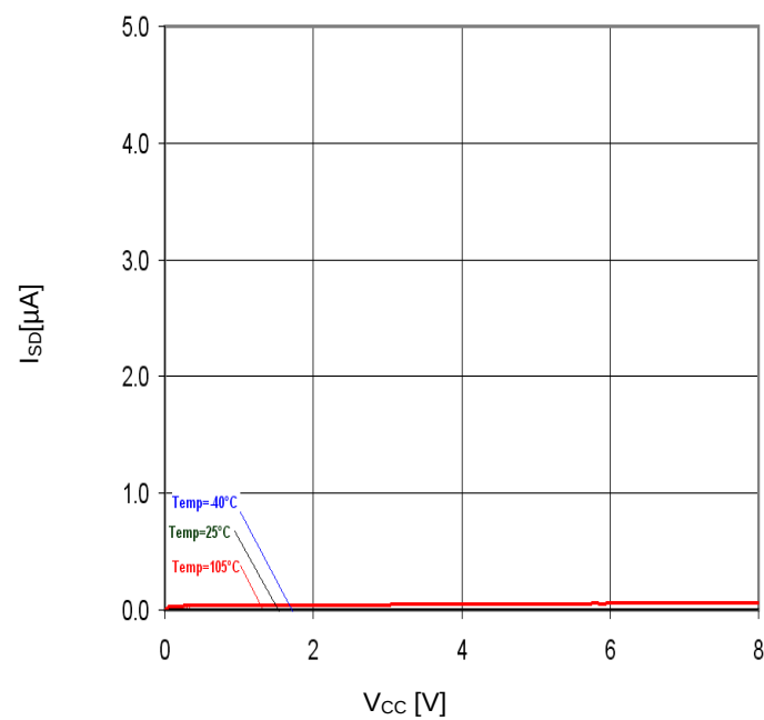
Figure 26. V CC -I SD (V EN =0V)
