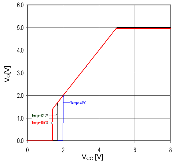
Figure 27. Vcc-Vo (Io=0mA)
