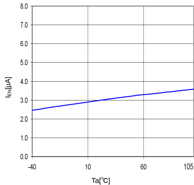
Figure 24. T a -I EN
