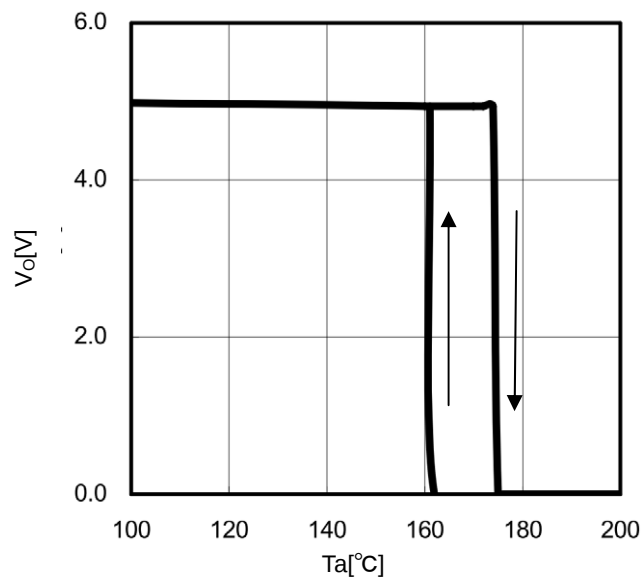
Figure 28. TSD (Io=0mA)
